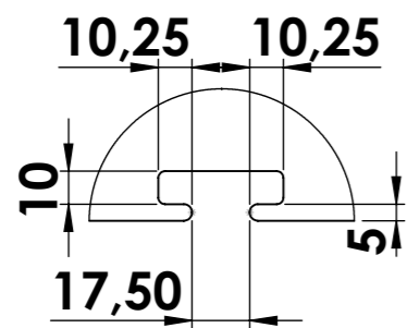
DÉTAIL A ECHELLE 2 : 5
